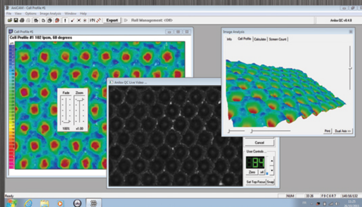
MODELISATION 3D (AVEC L'ANICAM) AVANT ET APRES DECOLMATAGE AVEC ARCHIVAGE DES DONNEES
